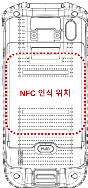
Figure 89 PM67 NFC 인식 위치
