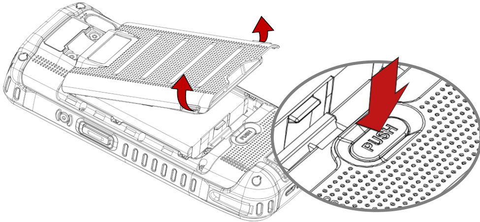
Figure 3 배터리 커버 열기
