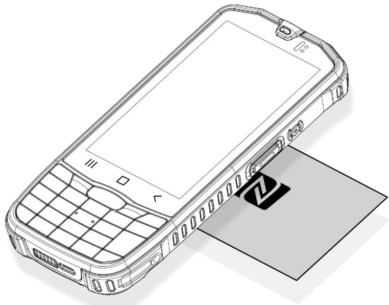
Figure 90 NFC 태그 인식
