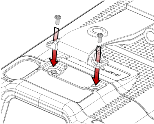
Figure 98 핸드 스트랩 장착하기 (브라켓)
