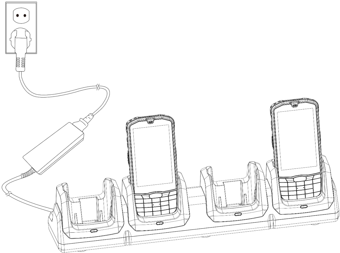
Figure 15 4SC 로 PM67 충전하기
