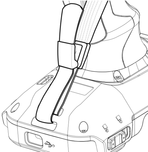
Figure 108 핸드 스트랩 연결하기 -3
