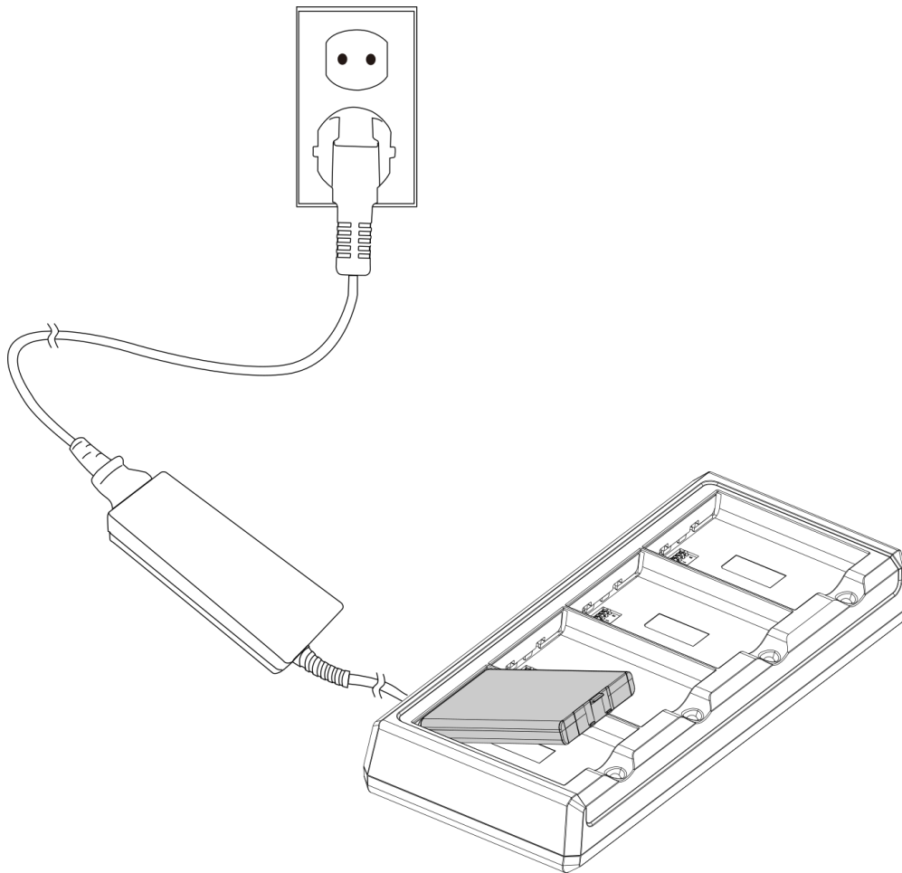
Figure 16 4SBC 로 PM67 배터리 충전하기
