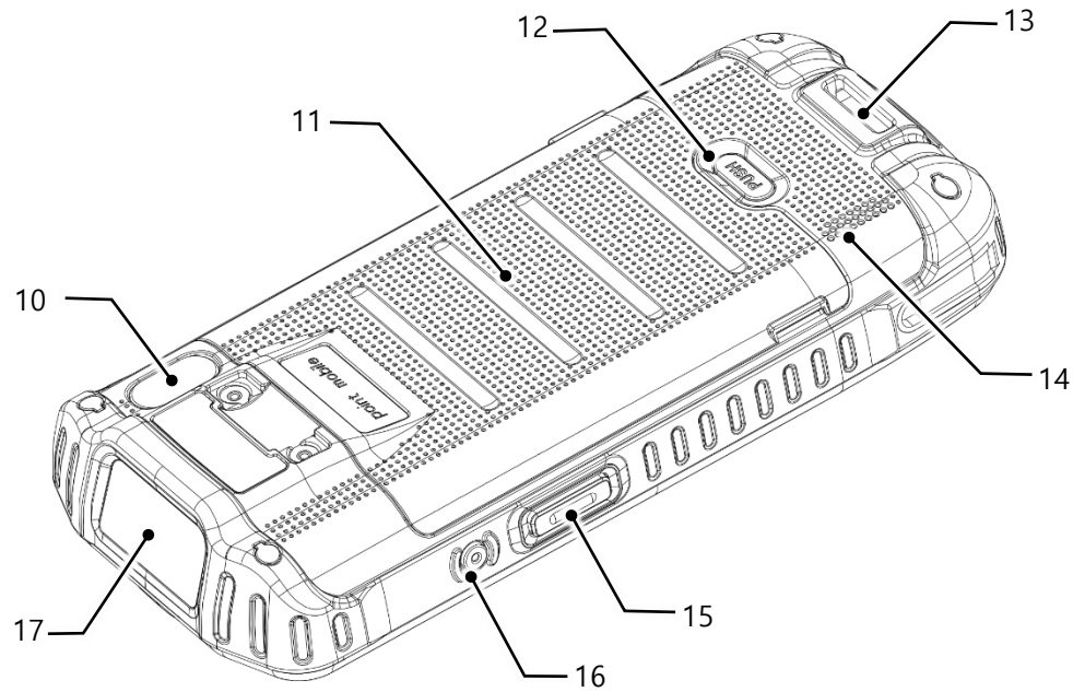
Figure 2 PM67 후면
