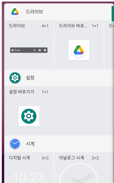
Figure 31 위젯 목록
