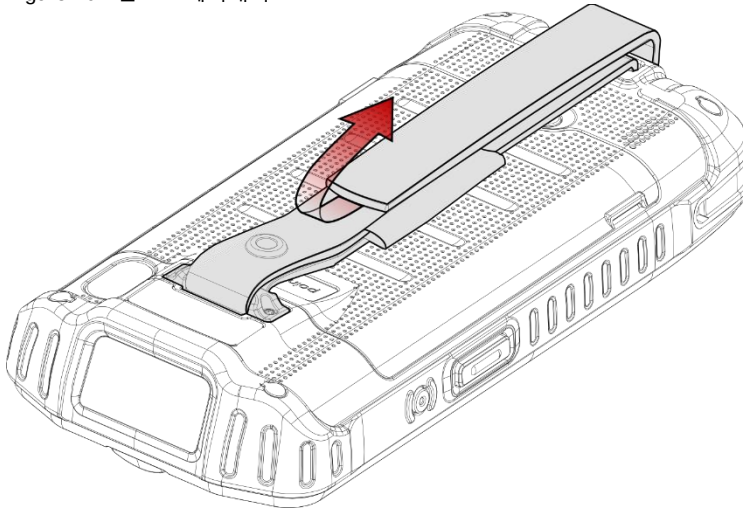
Figure 101 벨크로 떼어내기
