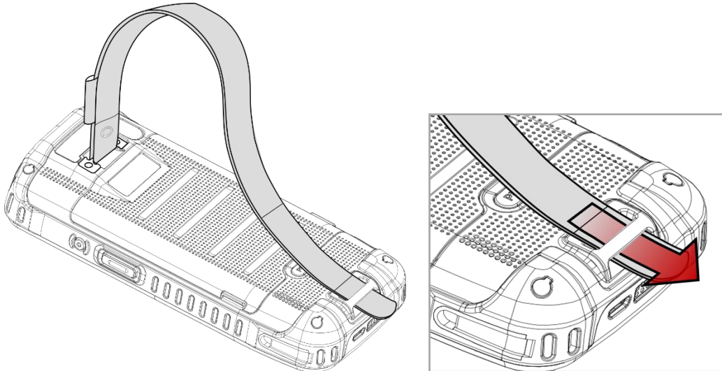
Figure 99 핸드 스트랩 연결부에 끼우기
