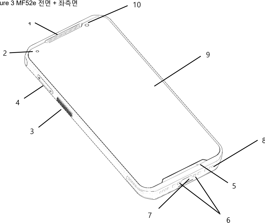
Figure 3 MF52e 전면 + 좌측면
