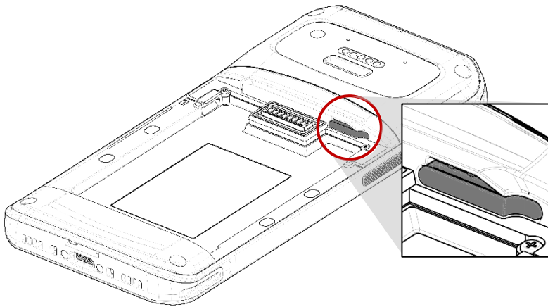
Figure 7 MF52e 카드 슬롯
