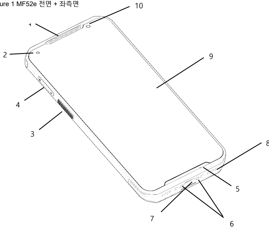
Figure 1 MF52e 전면 + 좌측면
