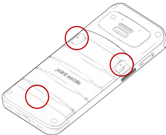
Figure 10 배터리 삽입하기 - 2
