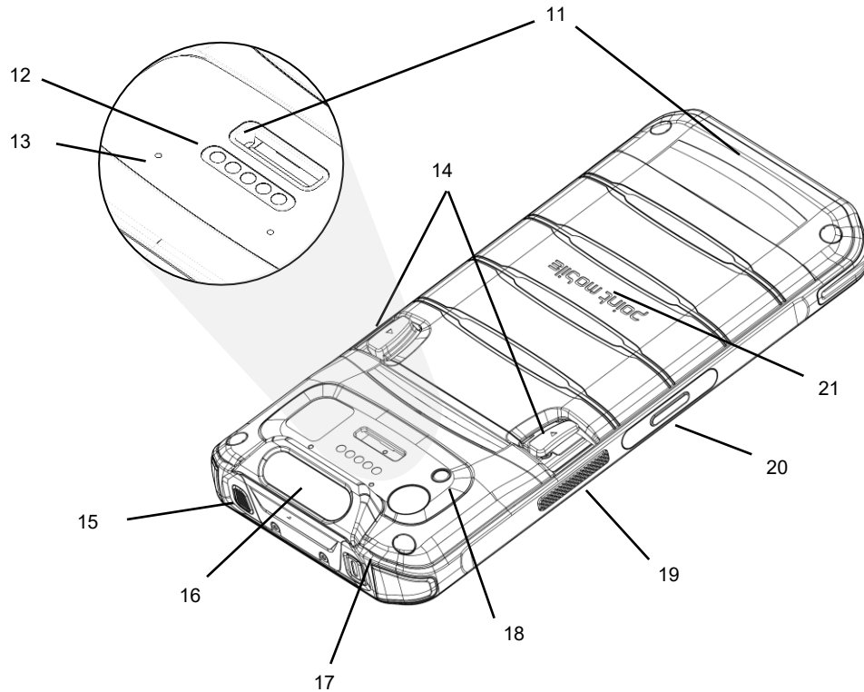
Figure 6 MF52e 후면 + 우측면
