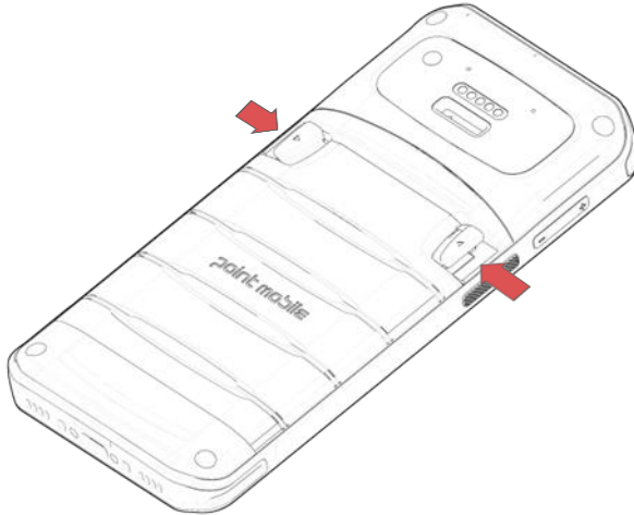
Figure 11 배터리 분리하기 - 1
