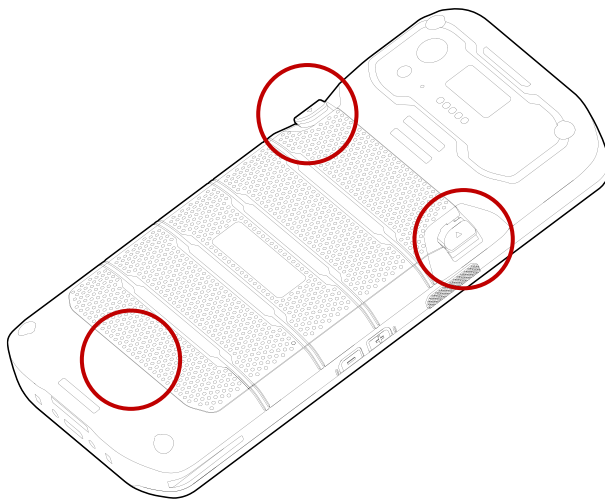
Figure 12 배터리 삽입하기 - 2
