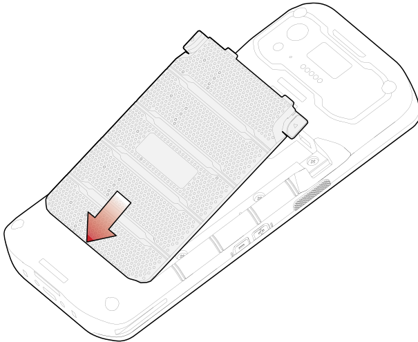
Figure 11 배터리 삽입하기 - 1
