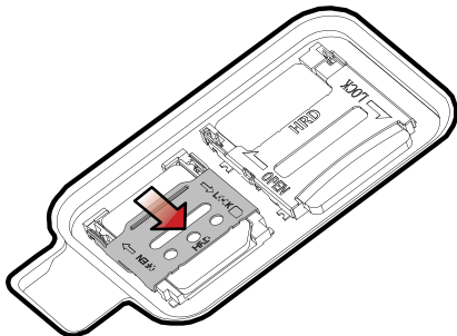
Figure 10 SIM 카드 슬롯 덮개 닫기
