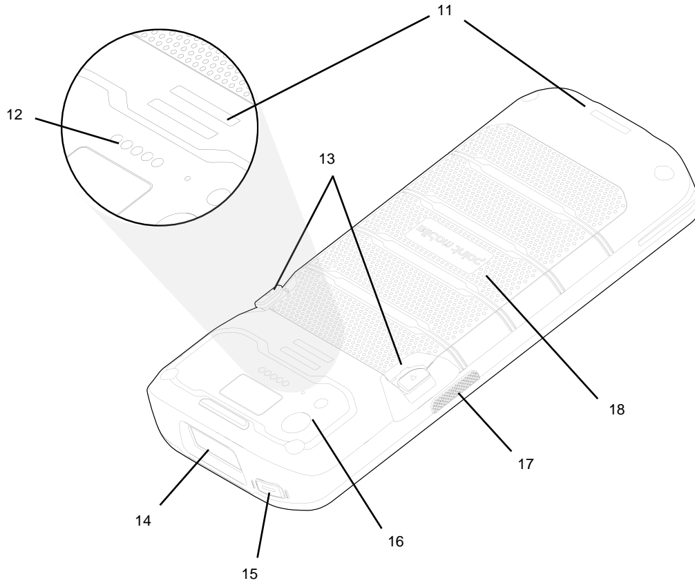
Figure 2 PM84 후면 + 우측면
