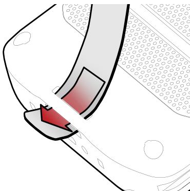
Figure 95 핸드 스트랩 연결하기 - 3
