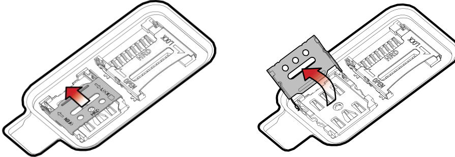
Figure 8 SIM 카드 슬롯 덮개 열기
