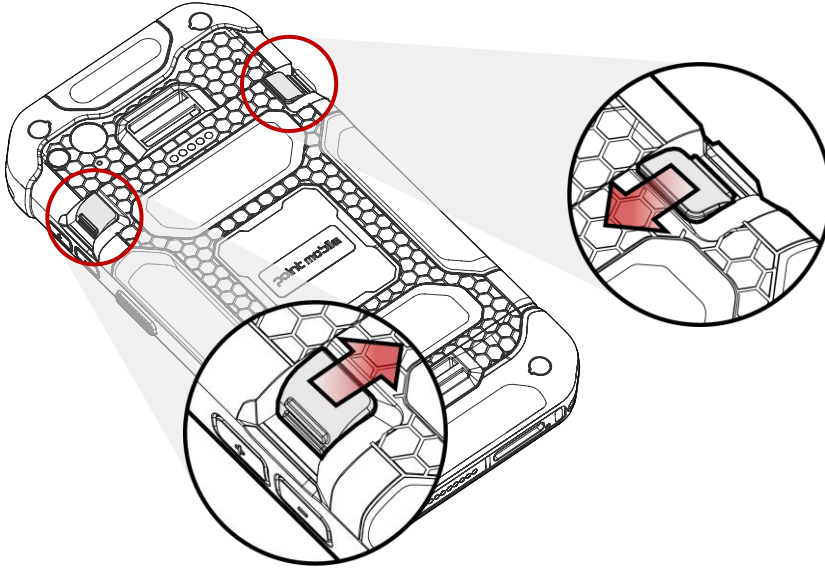
Figure 16 배터리 분리하기 - 1
