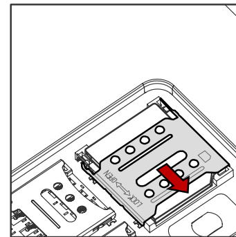
Figure 13 SAM 카드 슬롯 덮개 닫기
