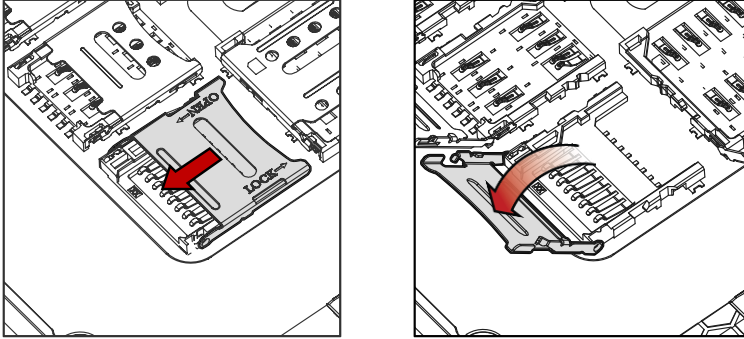
Figure 5 SD 카드 슬롯 덮개 열기
