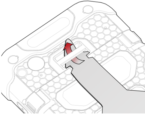
Figure 95 핸드 스트랩 연결하기_1
