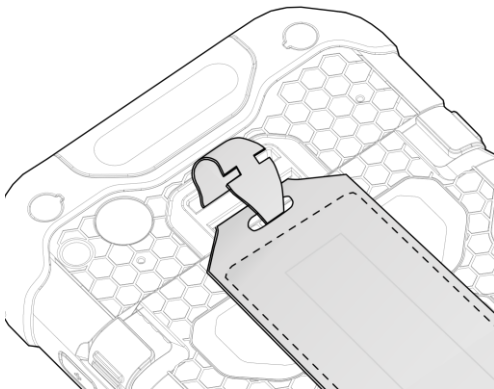
Figure 96 핸드 스트랩 연결하기_2
