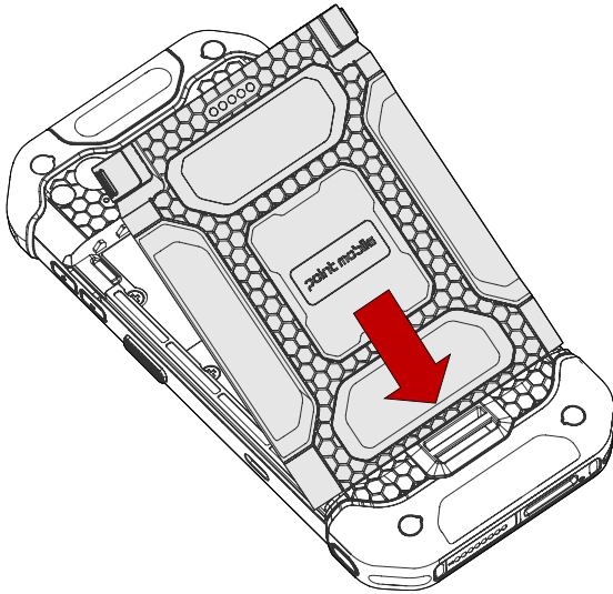
Figure 14 배터리 삽입하기 - 1
