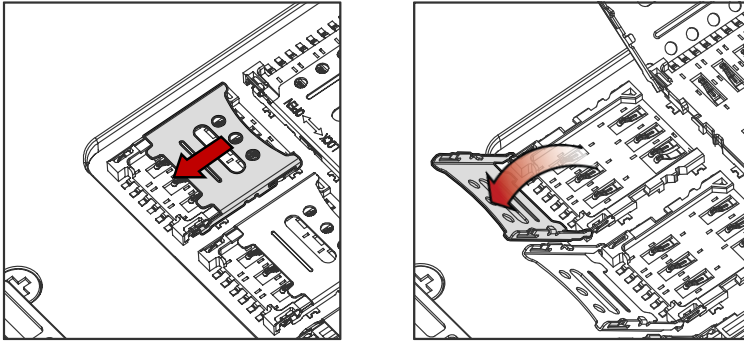
Figure 8 SIM 카드 슬롯 덮개 열기
