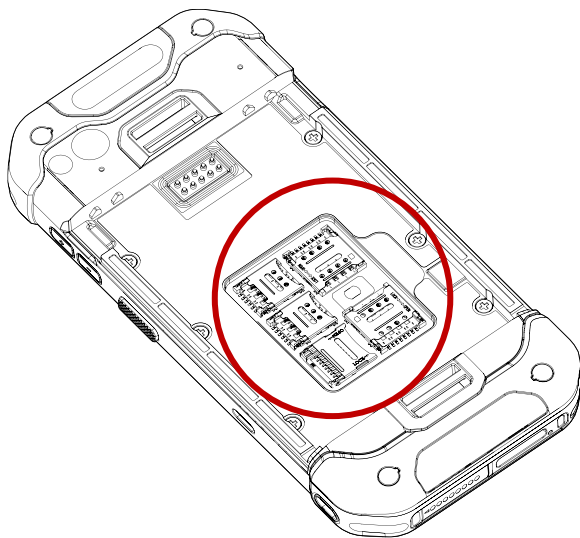
Figure 3 PM86 카드 슬롯
