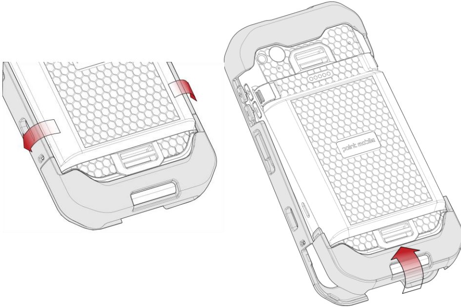
Figure 102 러기드 부트 분리하기_1
