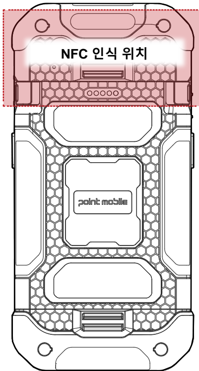
Figure 86 PM86 NFC 인식 위치
