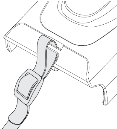
Figure 108 건 핸들 - 핸드 스트랩 연결하기_2
