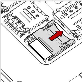
Figure 7 SD 카드 슬롯 덮개 닫기
