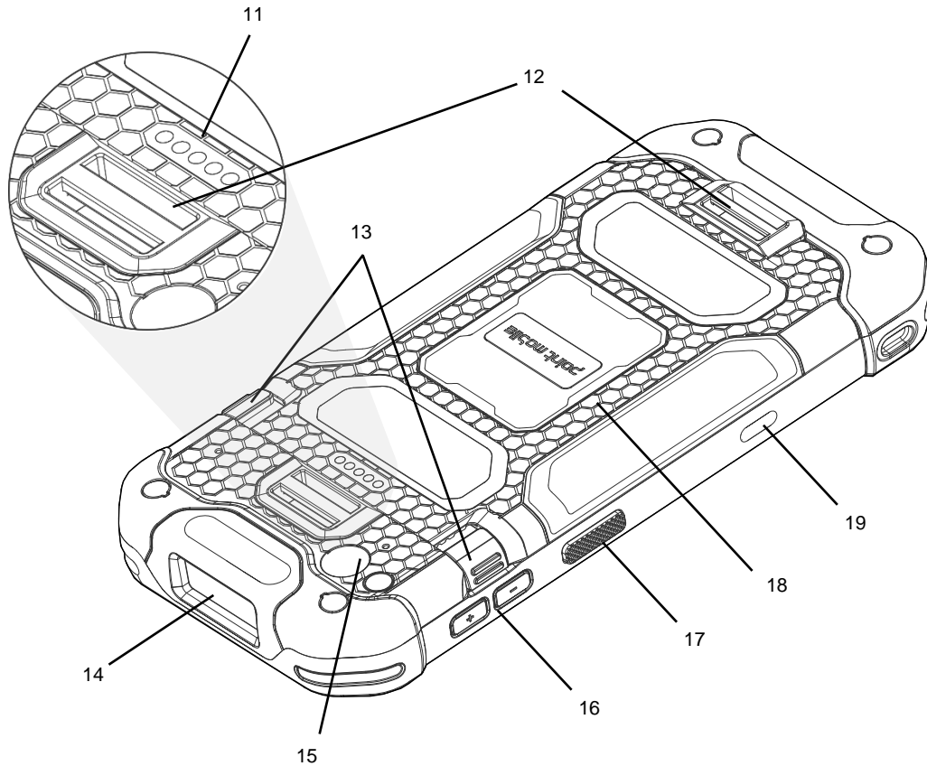
Figure 2 PM86 후면 + 우측면
