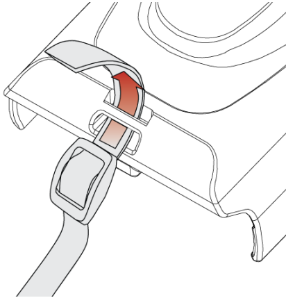
Figure 107 건 핸들 - 핸드 스트랩 연결하기_1
