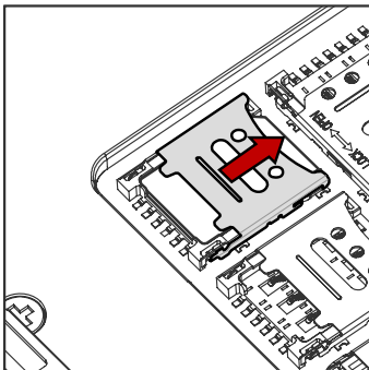
Figure 10 SIM 카드 슬롯 덮개 닫기
