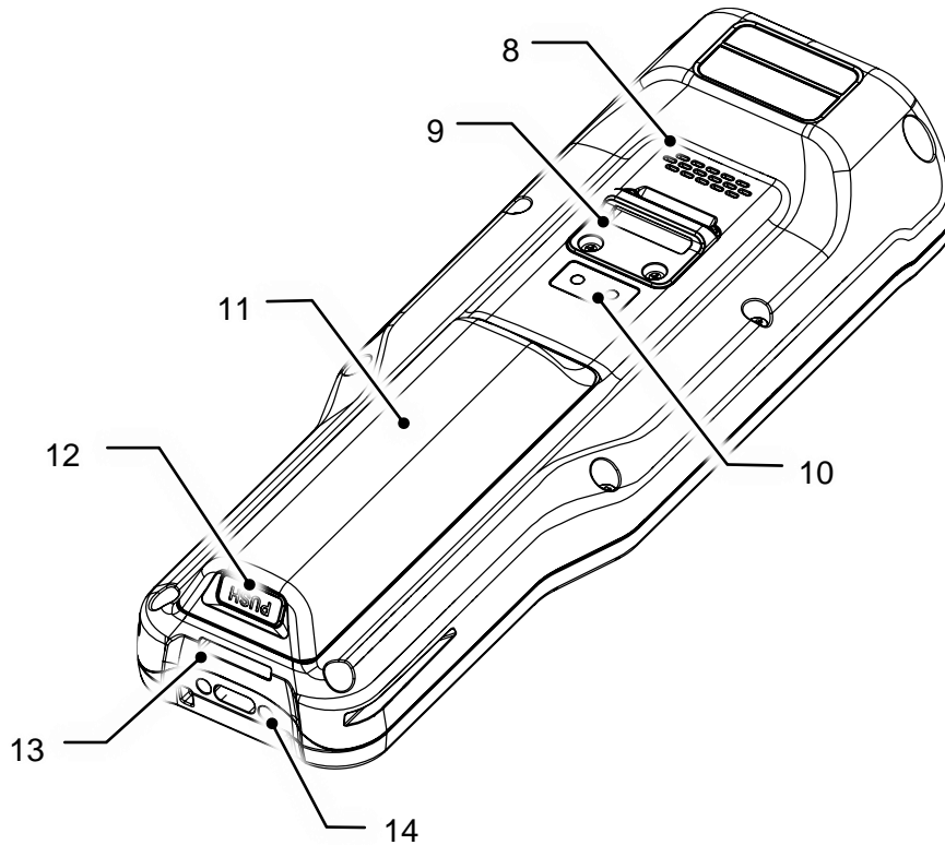
Figure 2 PM351 후면
