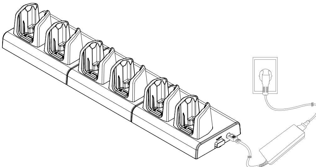
Figure 91 웨어 크래들(6SC)
